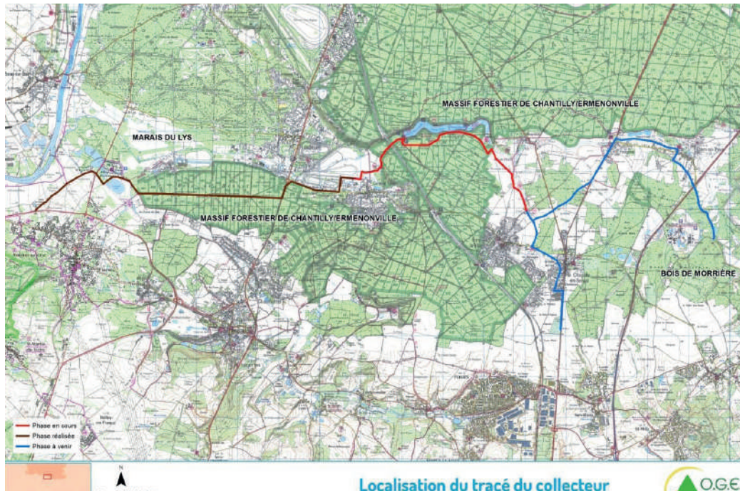
LOCALISATION DU TRACÉ DU COLLECTEUR DE LA VALLÉE DE LA THÈVE 2015 ET 2016
