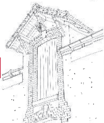
Lucarne à engranger engagée dans le toit, pour accès à l'étage dit "à encuvement"
